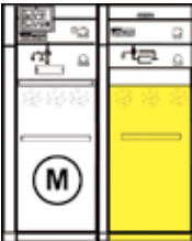
(M) 表示断路器功能单元加装了电动操作机构。
