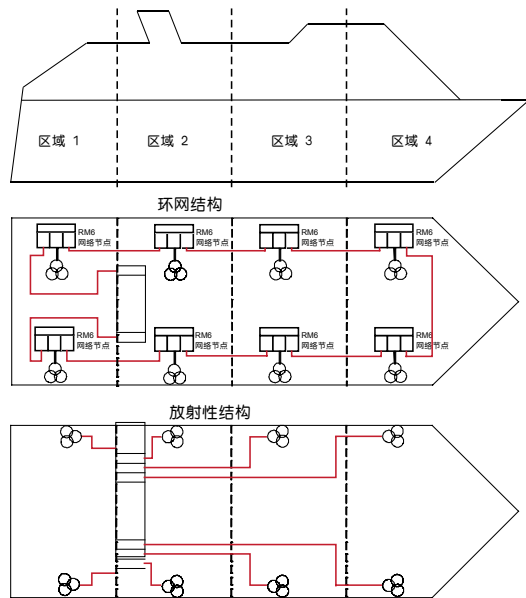
船用电配网结构举例
