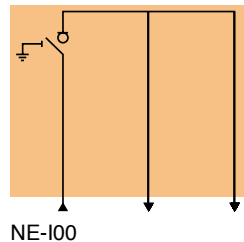
不可扩展的开关柜
