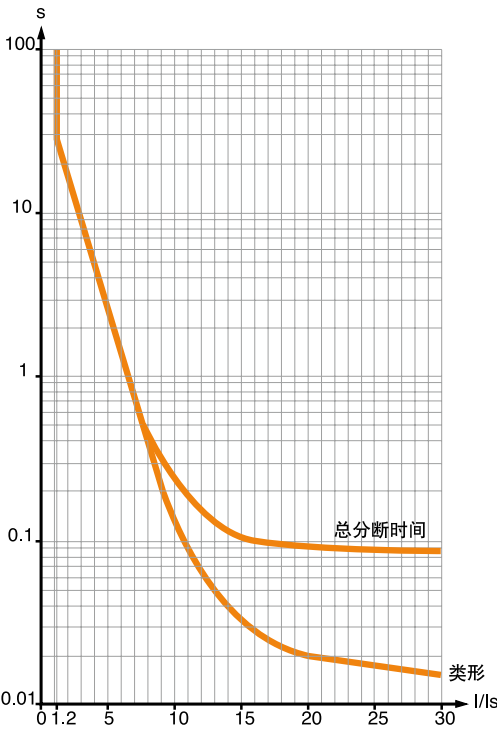
曲线表示继电器延时时间，分断时间应再加上70ms。
